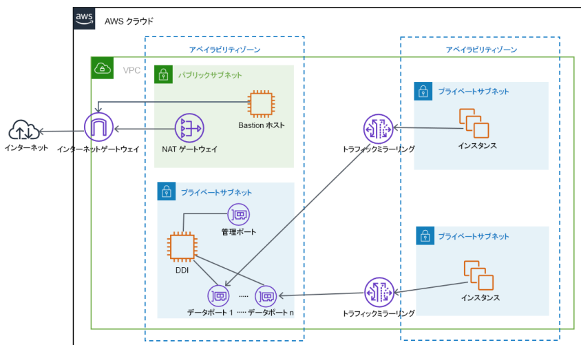
図 2-2. オプション 1: Deep Discovery Inspector 仮想アプライアンスをトラフィックミラーターゲットとして導入する
